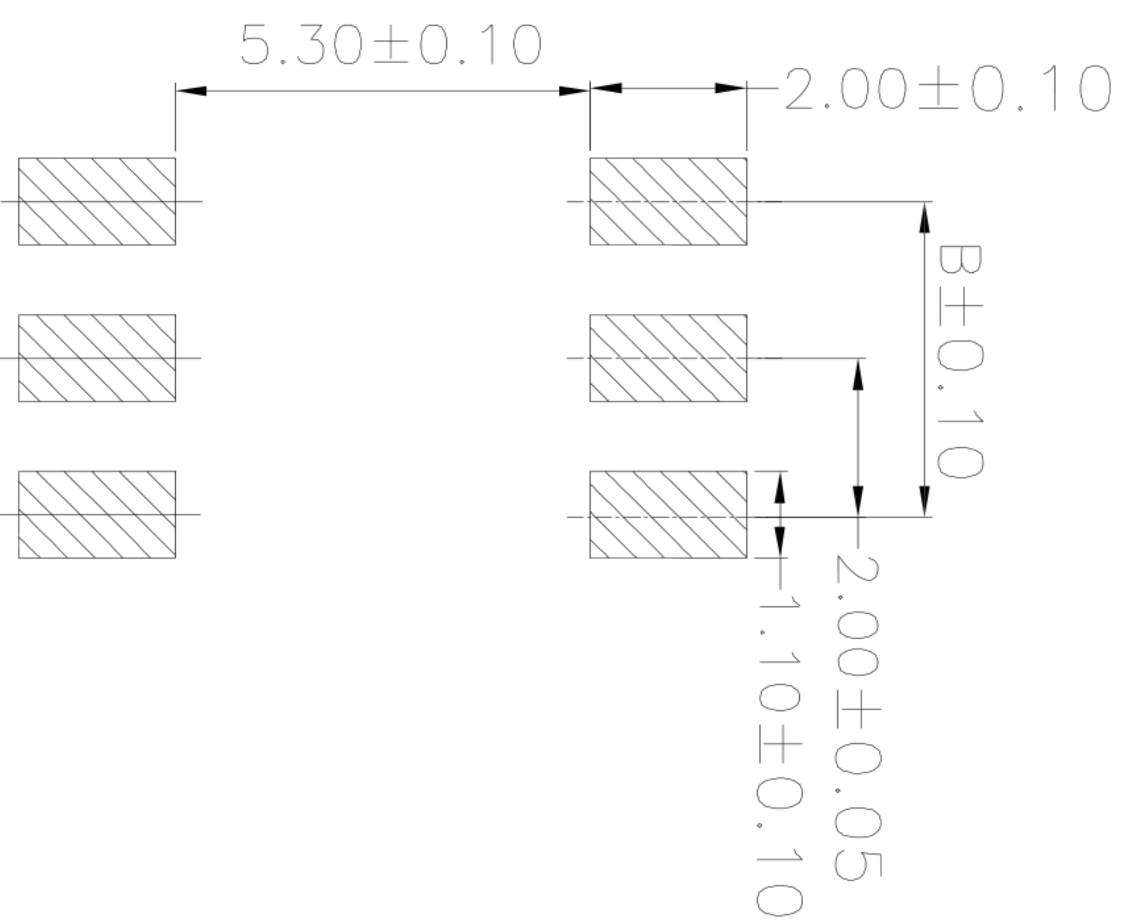
P.C.B LAYOUT
